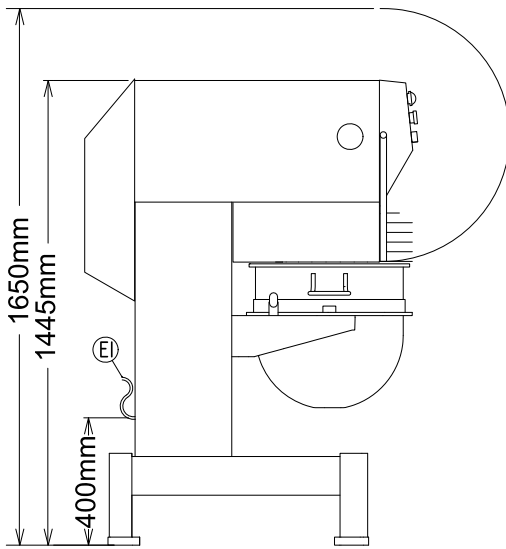
Oldalnézet
